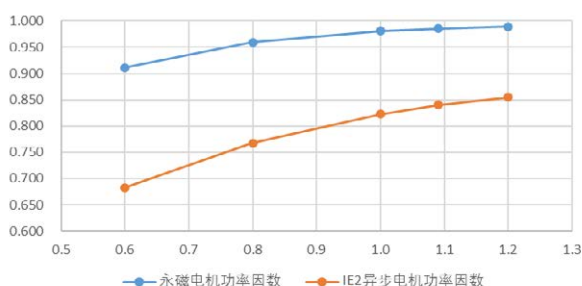
不同负载下电机功率因数变化曲线图 Power factor case
